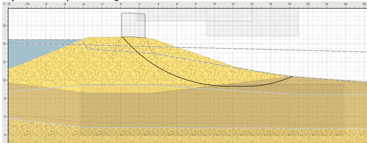
Glijvlak Plaxis – onverzadigd
