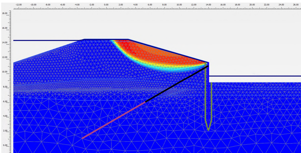
Figuur 17-5: DD265+30 – Maatgevend bezwijkmechanisme bij 10 l/s/m in de verzadigde situatie
